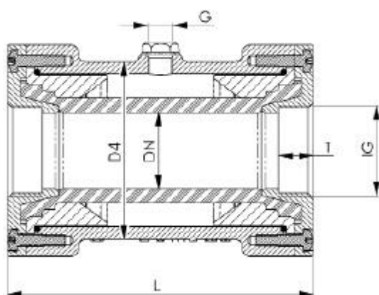
DN10 - DN15
